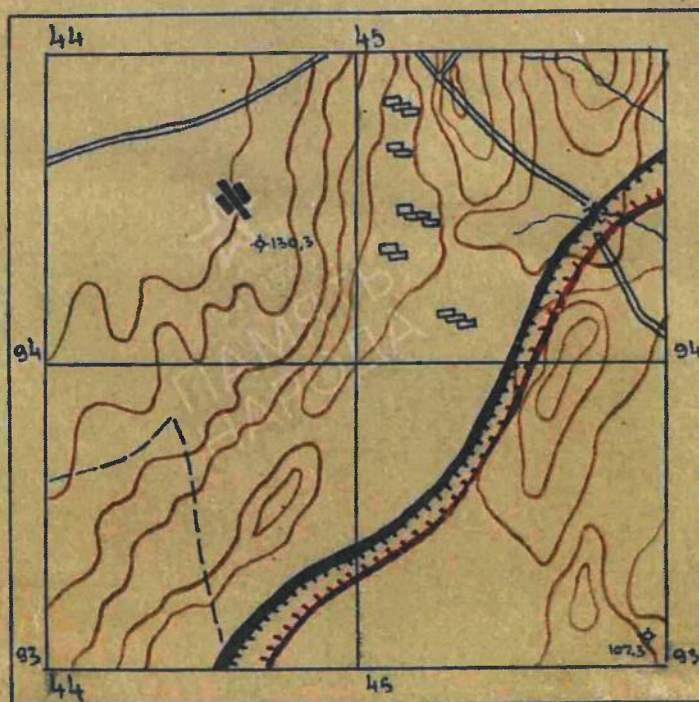
схема расположения засеченной 75мм. пушки пр-ка.
